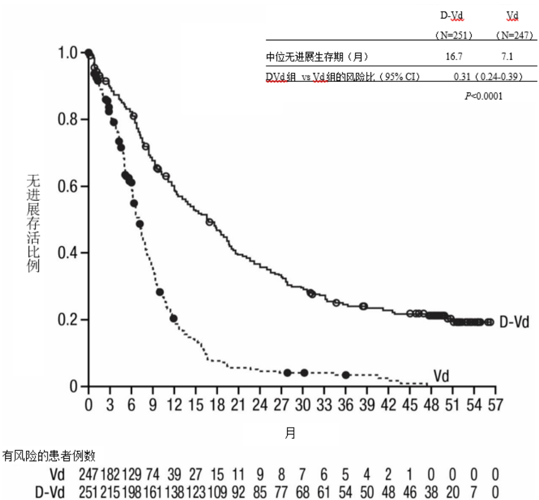
图 7： 研究 MMY3004 的 PFS Kaplan-Meier 曲线
